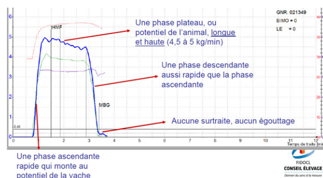
Courbe de traite idéale
