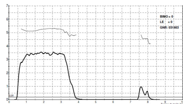
Courbe d'éjection du lait en L/min avec surtaite
